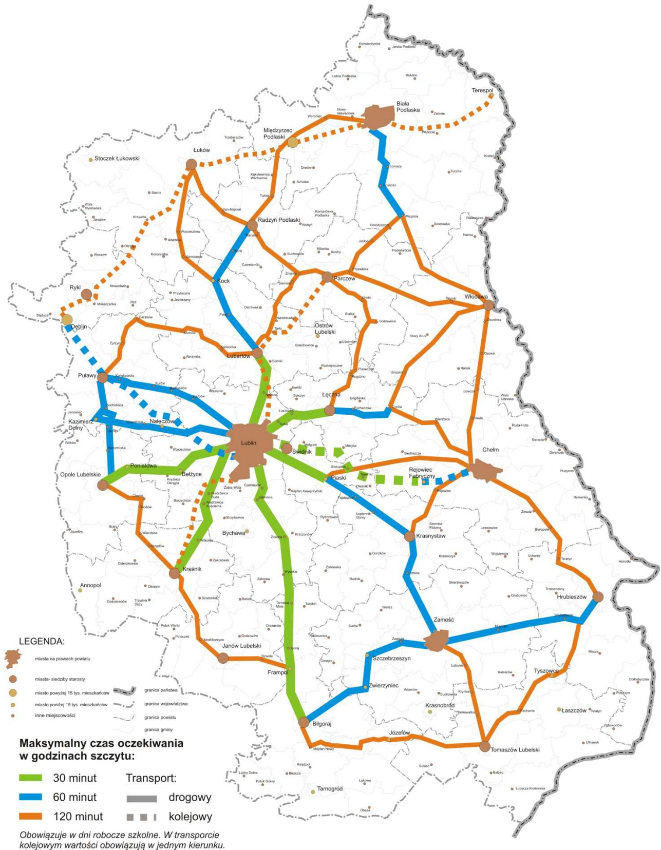
Rys. 7.2. Kategoryzacja linii komunikacyjnych w transporcie drogowym oraz na gwarantowanych przez Województwo Lubelskie połączeń w transporcie kolejowym na przykładzie godzin szczytów komunikacyjnych w dni robocze szkolne. Źródło: opracowanie własne.
