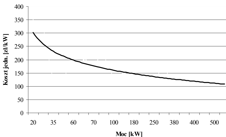
Rys. 8 Jednostkowe koszty zakupu kotłów na słomę
