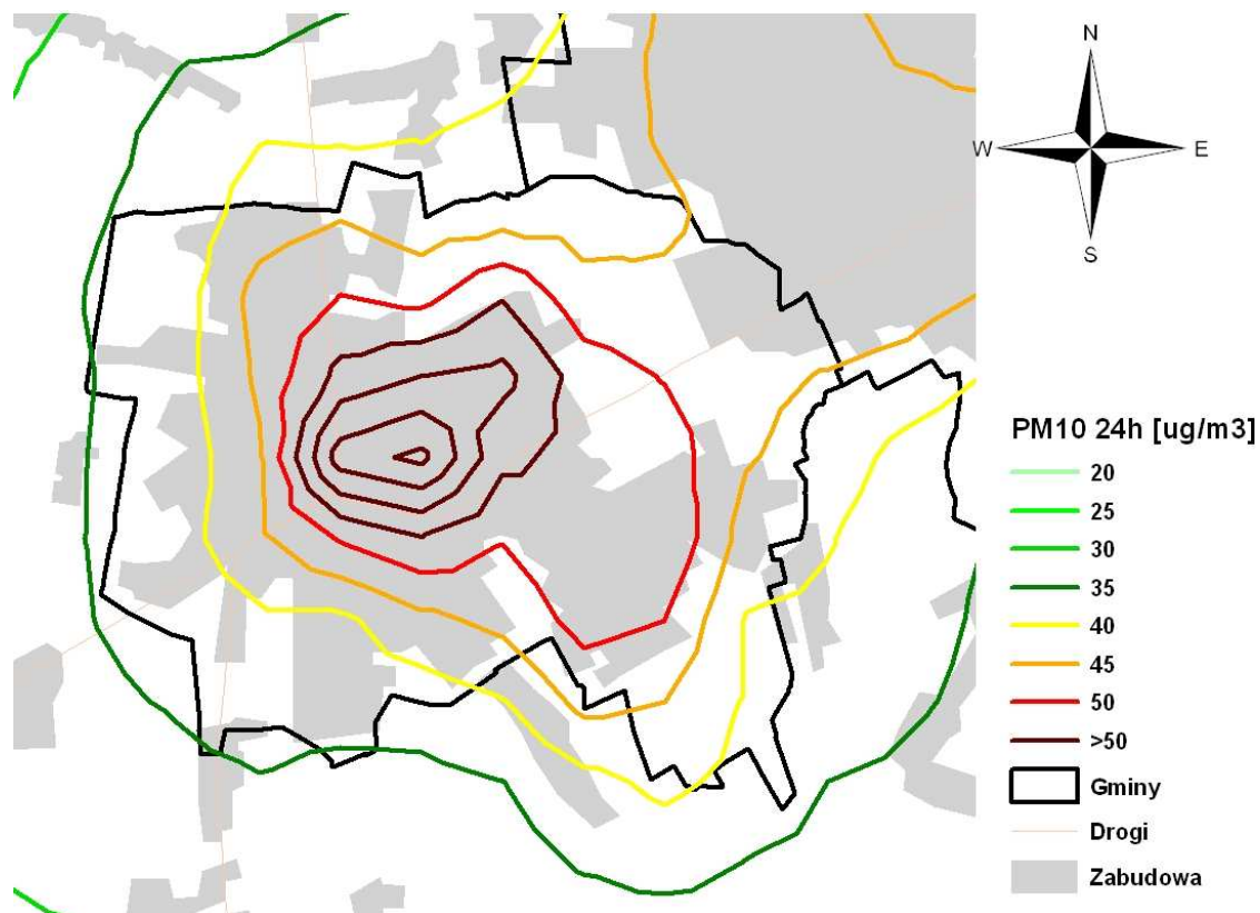
Rysunek 3.37 Rozkład stężeń pyłu zawieszonego PM10 o okresie uśredniania wyników pomiarów 24 godziny na terenie Grodziska Mazowieckiego w 2005 roku
