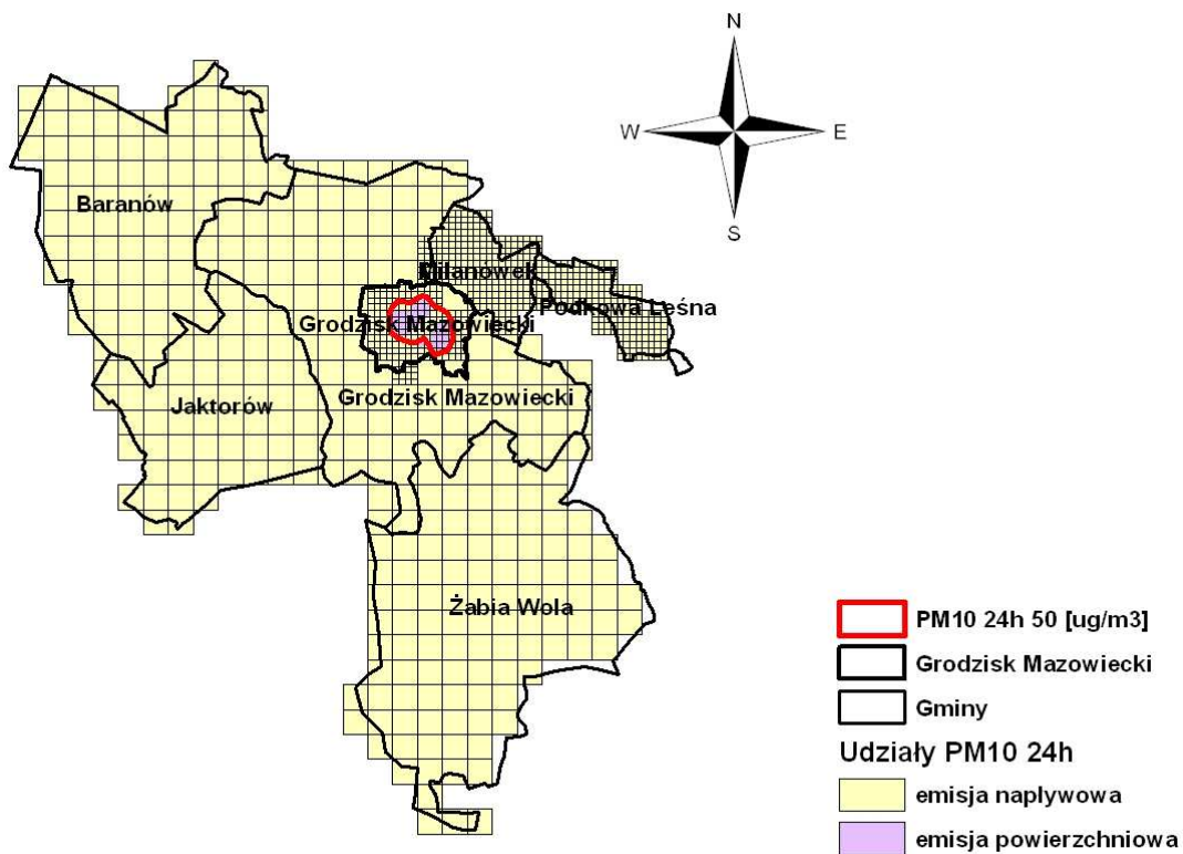
Rysunek 3.40 Udział typów emisji w stężeniach pyłu zawieszonego PM10 o okresie uśredniania wyników pomiarów 24 godziny w receptorach na obszarze powiatu grodzkiego
