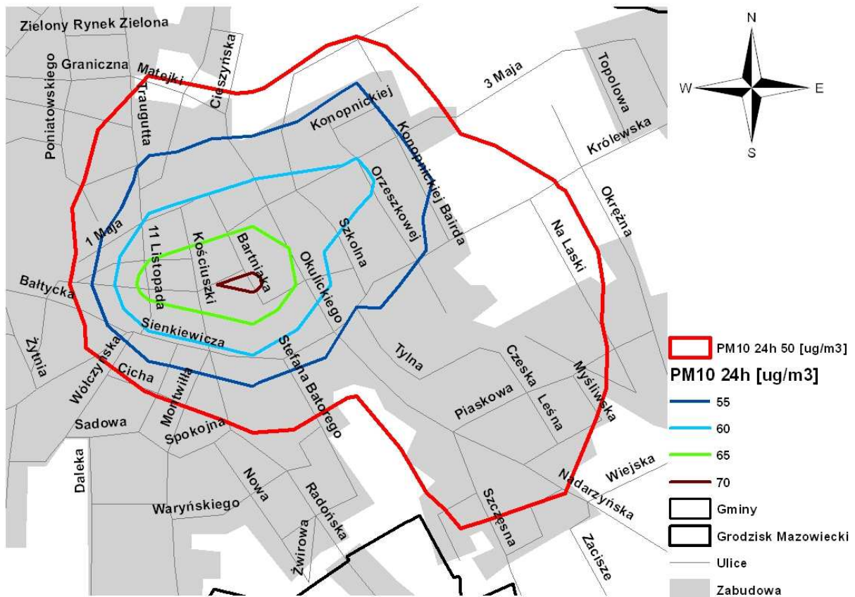
Rysunek 4.1 Obszar Grodziska Mazowieckiego w obrębie izoliny 50 µg/m 3 , stężenia pyłu zawieszonego PM10 o okresie uśredniania wyników pomiarów 24 godziny pochodzące od całości emisji w 2005 roku
