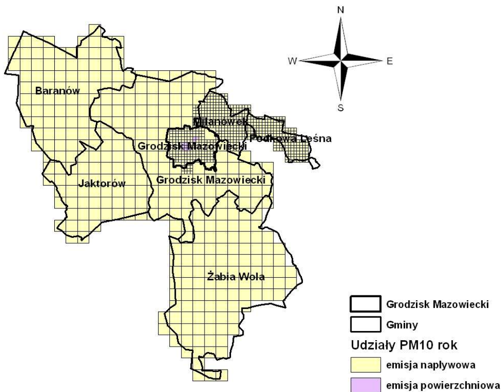
Rysunek 3.41 Udział typów emisji w stężeniach pyłu zawieszonego PM10 o okresie uśredniania wyników pomiarów rok kalendarzowy w receptorach na obszarze powiatu grodzkiego
