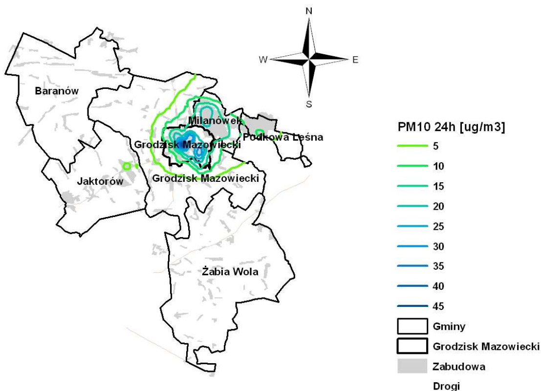
Rysunek 3.28 Rozkład stężeń pyłu zawieszonego PM10 o okresie uśredniania wyników pomiarów 24 godziny pochodzących od emisji powierzchniowej na terenie powiatu grodziskiego w 2005 roku
