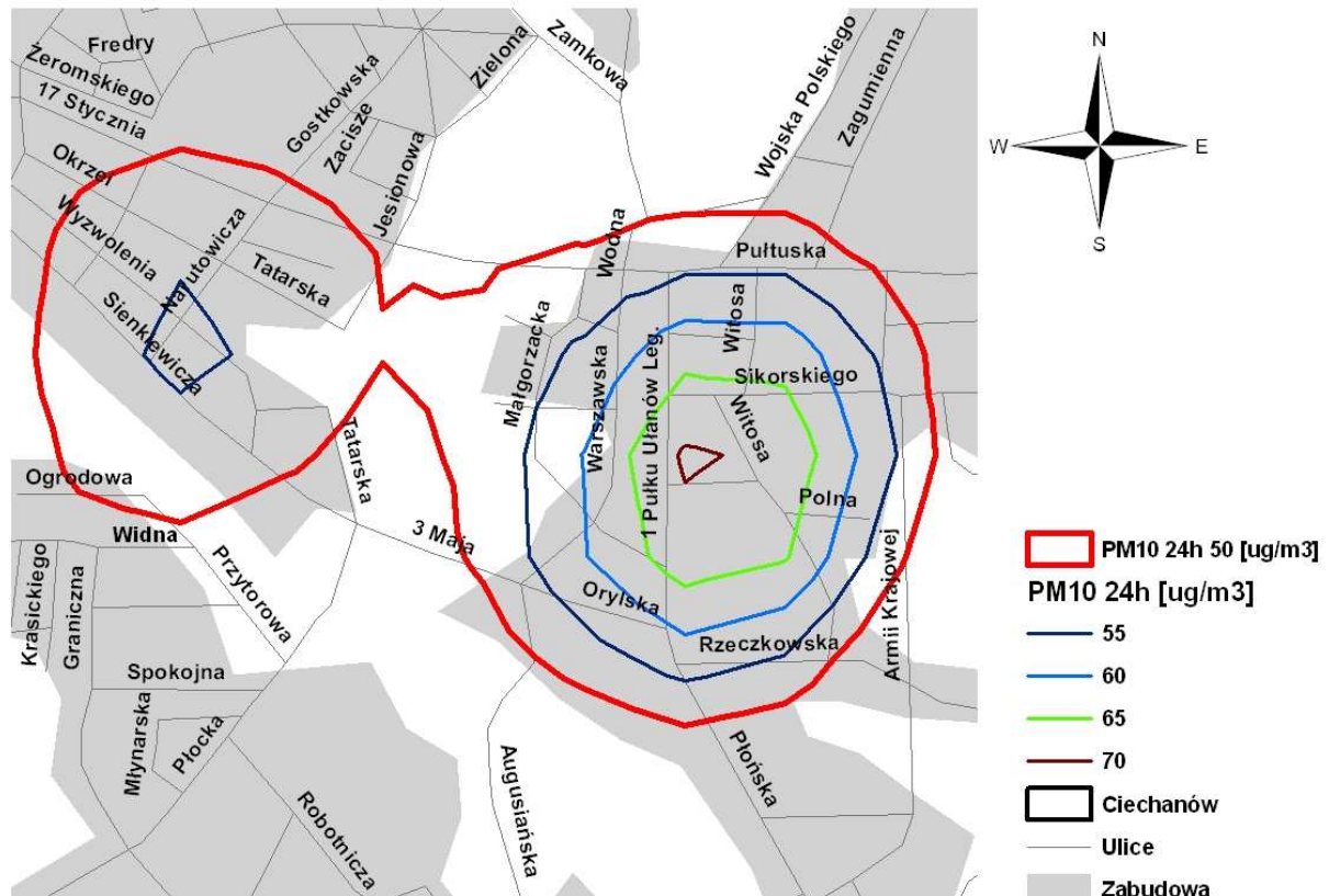
Rysunek 4.1 Obszar Ciechanowa w obrębie izoliny 50 \mu\text{g}/\text{m}^3 , stężenia pyłu zawieszonego PM10 o okresie uśredniania wyników pomiarów 24 godziny pochodzące od całości emisji w 2005 roku
