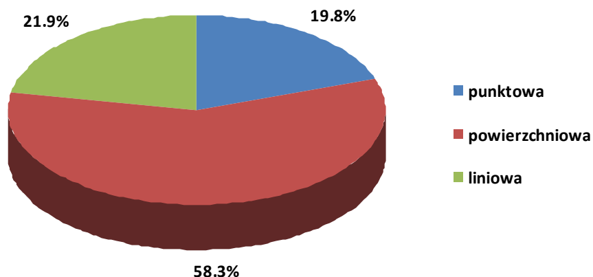
Rysunek 3.20 Udział procentowy poszczególnych typów źródeł emisji w całości zinwentaryzowanej emisji pyłu zawieszonego PM10 na terenie Legionowa w 2006 roku
