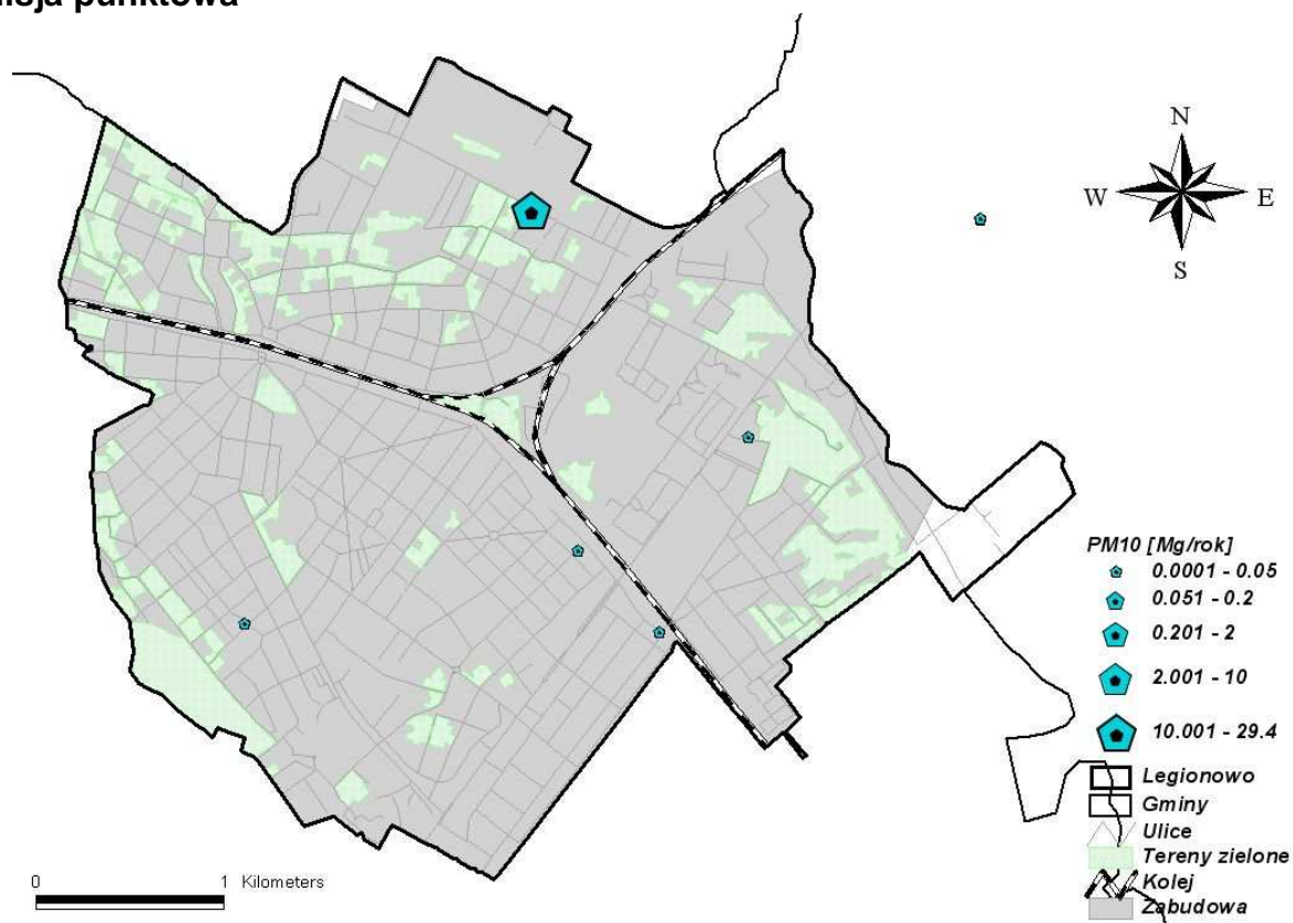
Rysunek 3.21 Emisja punktowa pyłu zawieszonego PM10 z emitorów punktowych w Legionowie w 2006 roku
