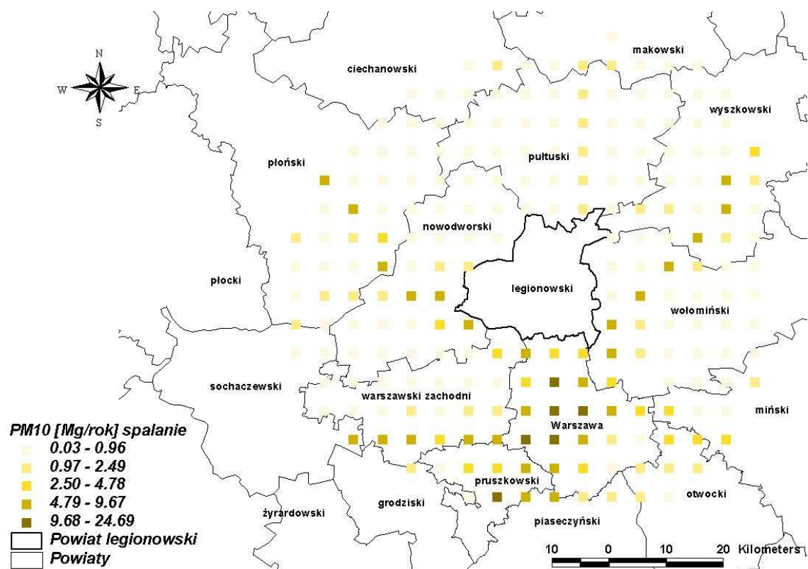
Rysunek 3.7 Emisja pyłu zawieszonego PM10 ze spalania, ze źródeł liniowych zlokalizowanych w pasie 30 km od powiatu legionowskiego w 2006 roku
