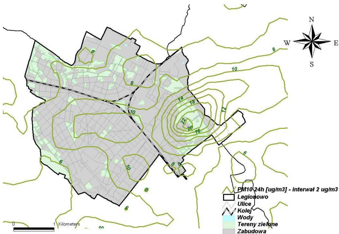
Rysunek 3.46 Rozkład stężeń pyłu zawieszonego PM10 o okresie uśredniania wyników pomiarów 24 godziny pochodzących od emisji powierzchniowej, w Legionowie w 2006 roku
